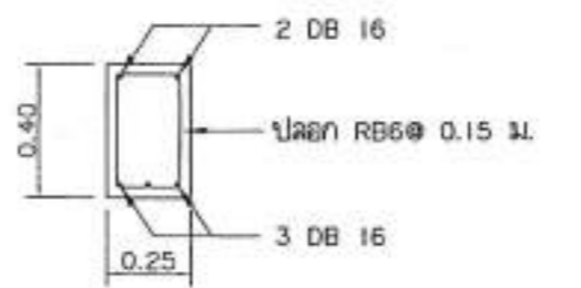
แบบขยายคาน B มาตราส่วน 1:25
