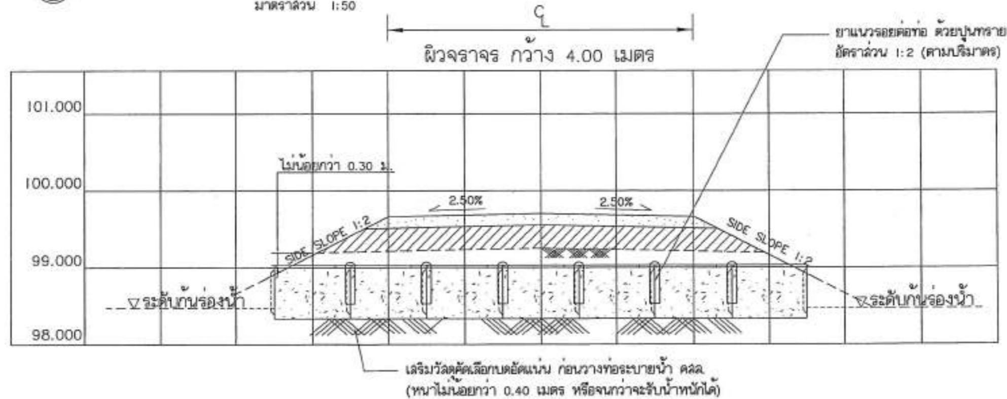
แสดงรูปตัดถนน ช่วง STA.ที่ฝังท่อระบายน้ำ คลล. ผิวจราจรกว้าง 4.00 เมตร (ขนาดท่อและจำนวนตามที่ระบุ)
