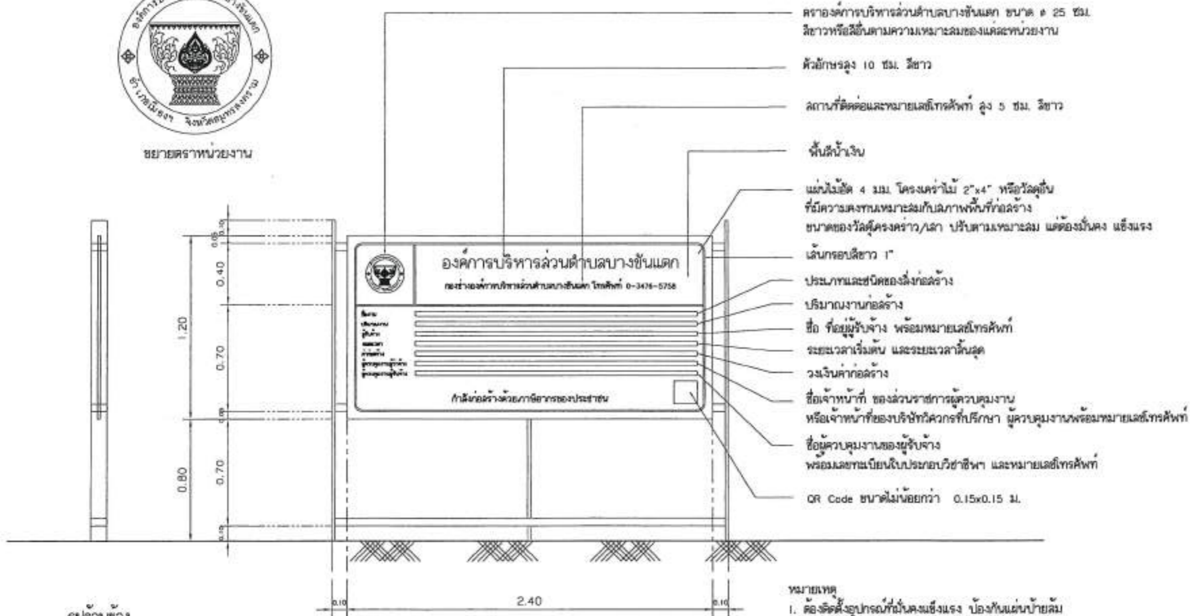
รูปด้านข้าง SCALE 1:25
