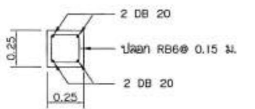
แบบขยายเสาตอมือ มาตราส่วน 1:25
