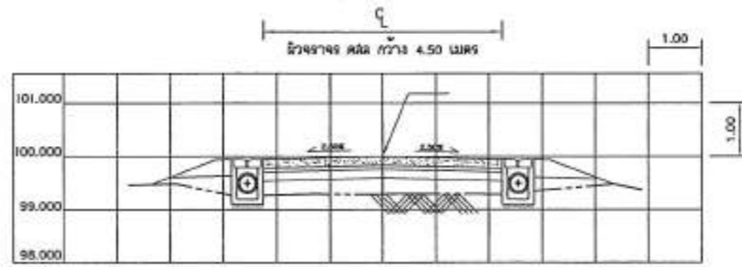
STA. 0+025 (แยกไปทางขวา)
