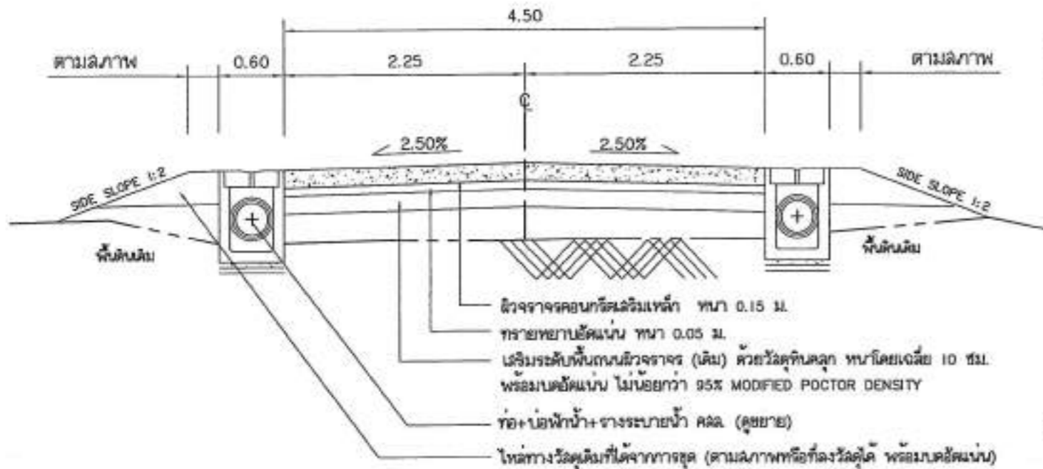
รูปตัดโครงสร้างทาง ช่วง 3 กม. ที่ 0+000-0+018.50 ช่วง 0+018.50-0+044 (ซ้ายทาง) และช่วง 0+018.50-0+039.50 (ขวาทาง)
