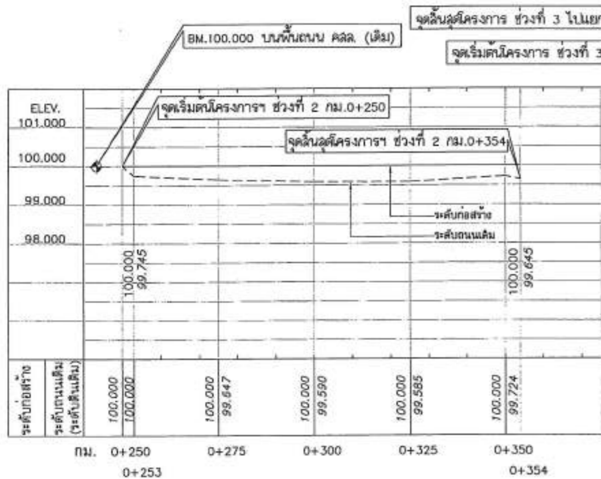
แสดงค่าระดับ ช่วงที่ 2 กม.ที่ 0+250-0+354 SCALE 1 : -
