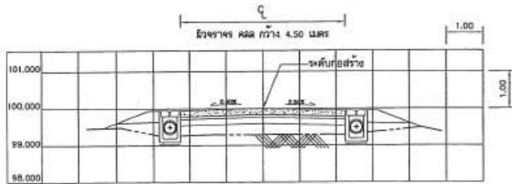
STA. 0+050
