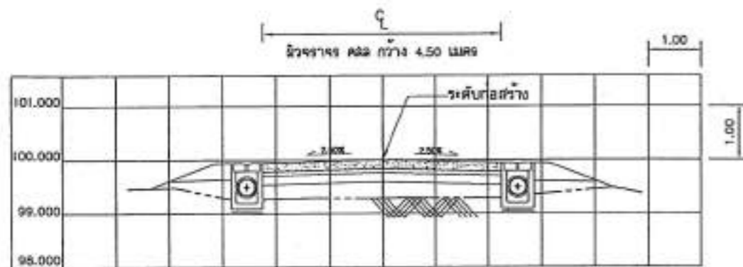
STA. 0+025 (แยกไปทางซ้าย)
