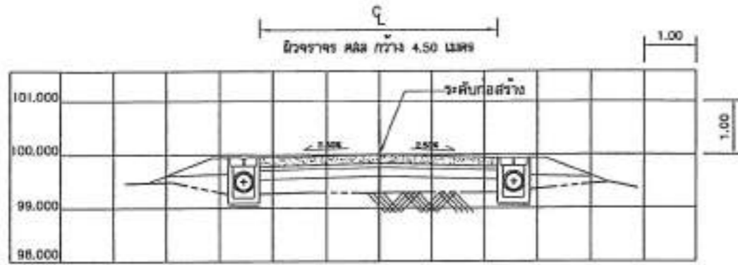
STA. 0+000
