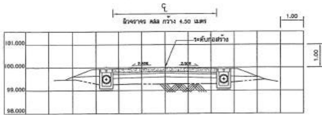
STA. 0+025
