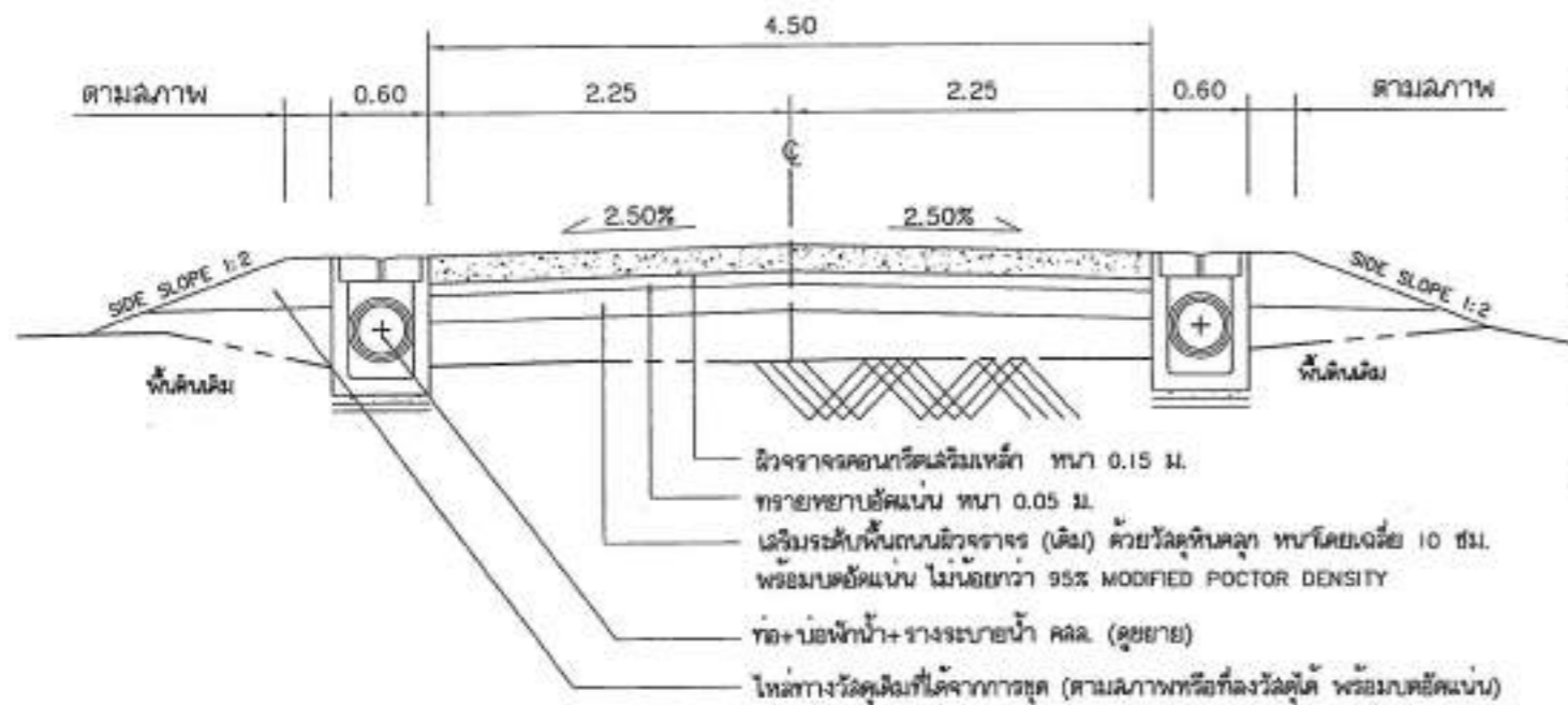
รูปตัดโครงสร้างทาง ช่วง ที่ 4 กม. ที่ 0+010-0+069 (แยกซ้าย)
