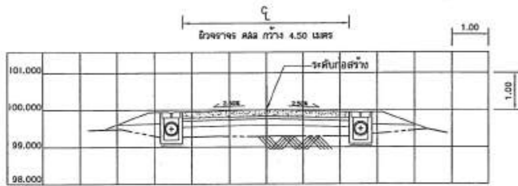
STA. 0+018.50
