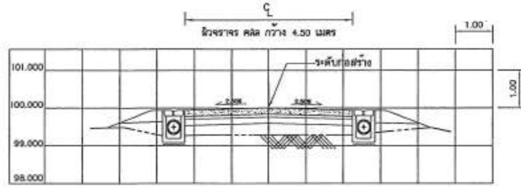
STA. 0+044 (แยกไปทางซ้าย)
