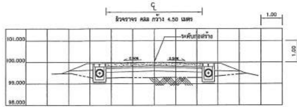
STA. 0+059
