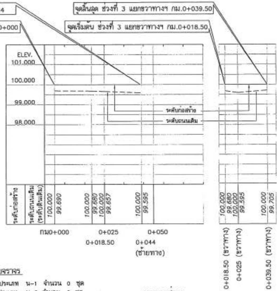
แสดงค่าระดับ ช่วง 3 กม.ที่ 0+000-0+018.50 ช่วง 0+018.50-0+0+44 (ซ้ายทาง) และช่วง 0+018.50-0+039.50 (ขวาทาง) SCALE 1 : -
