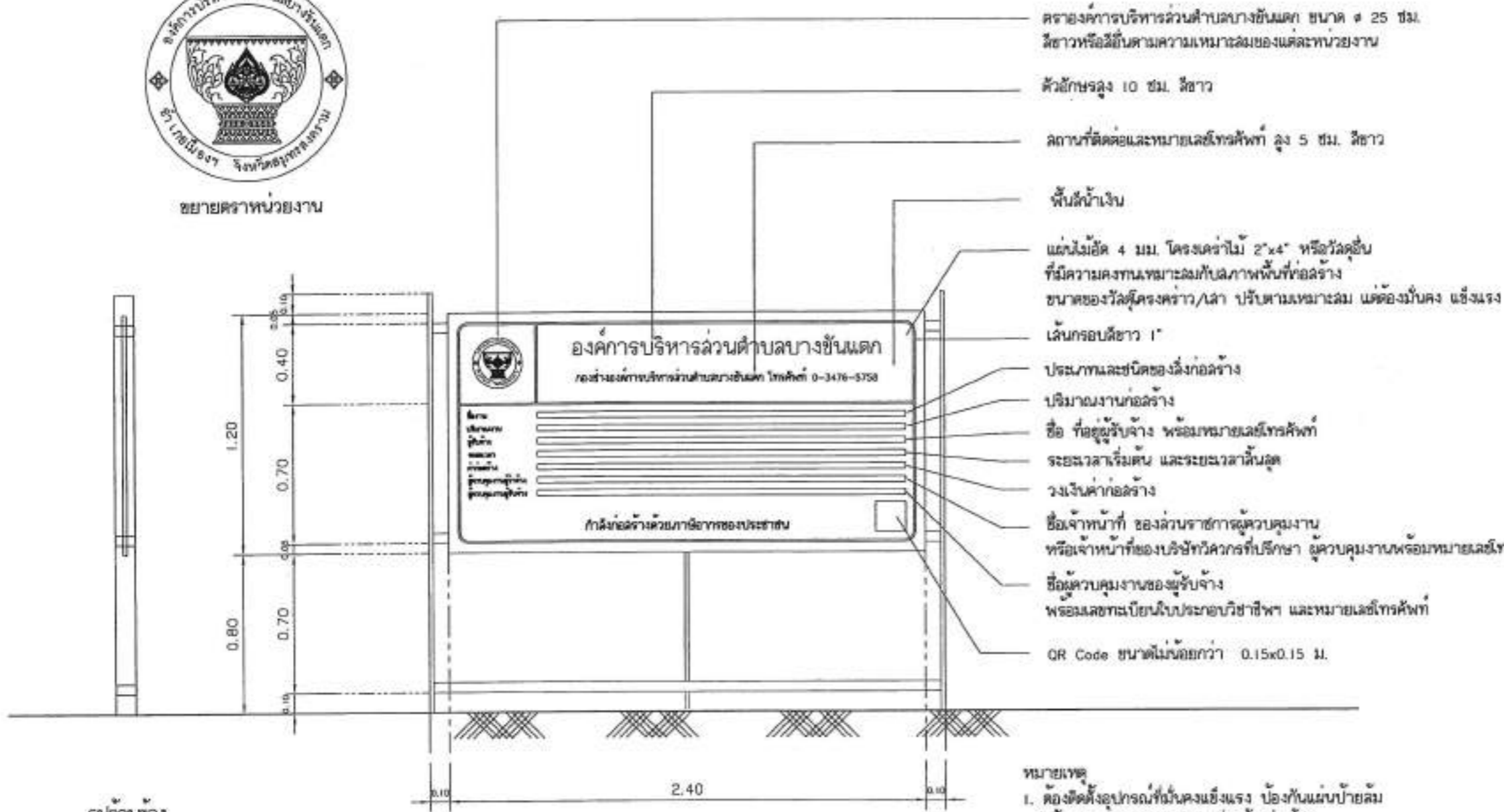
รูปด้านข้าง SCALE 1:25
