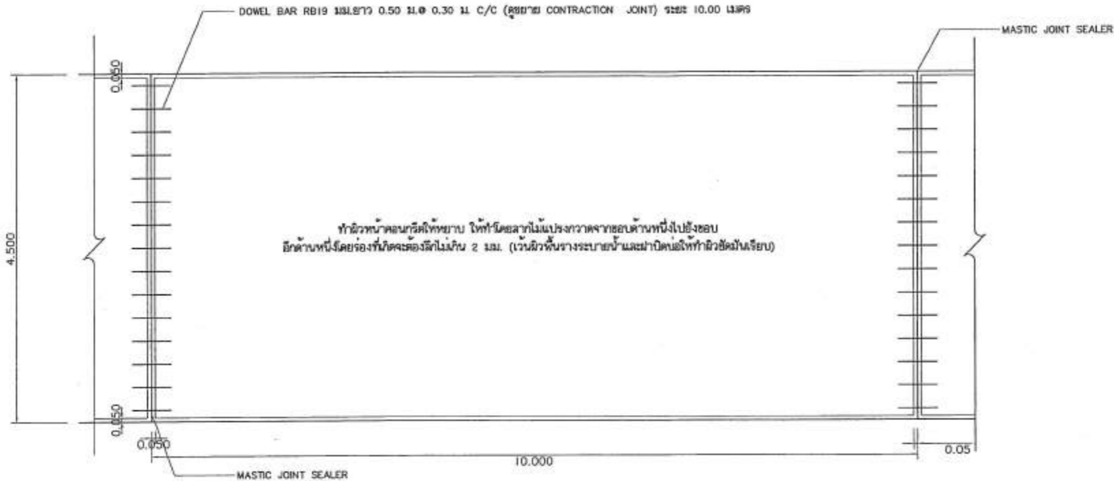
แปลนผิวจราจร คสล. SCALE 1:50
