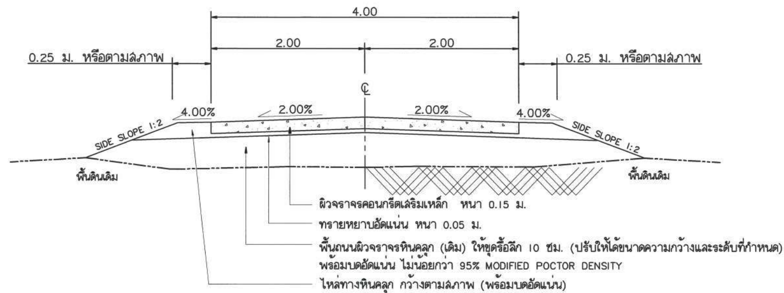
รูปตัดโครงสร้างทาง ช่วง กม.ที่ 0+000-0+350 และช่วง กม.ที่ 0+374-0+415 SCALE 1:50
